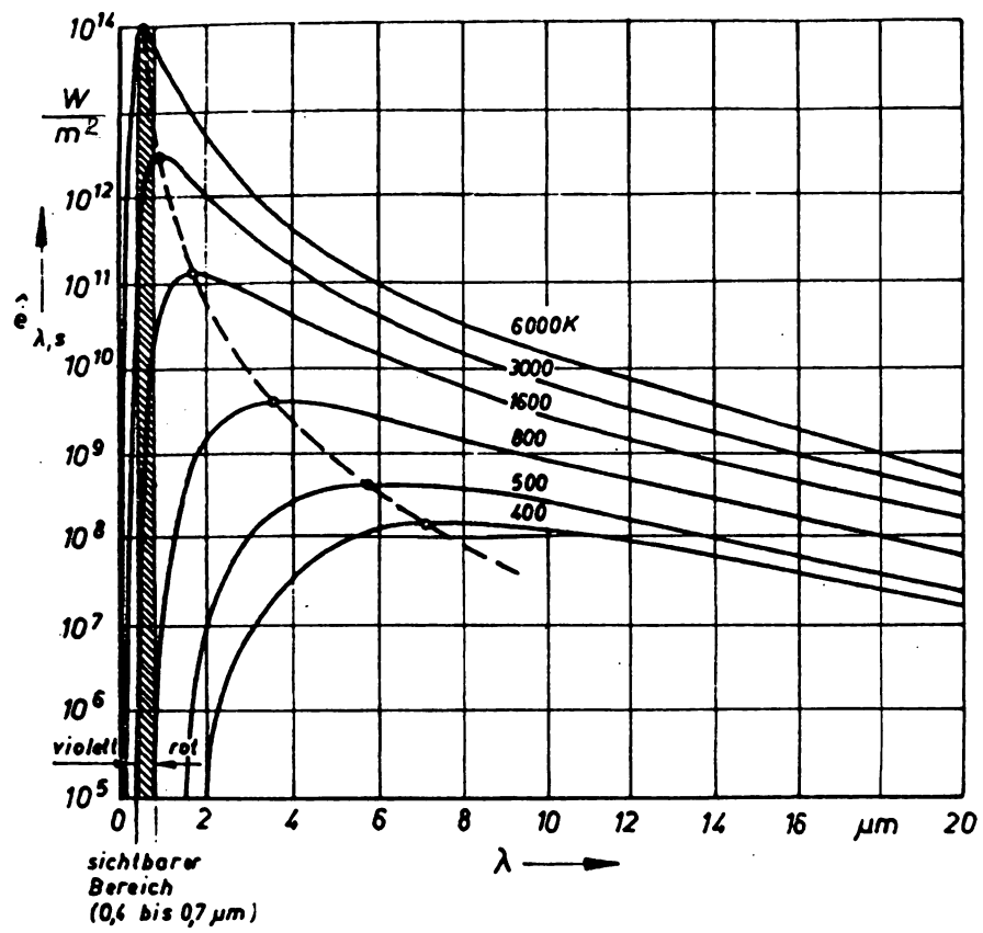
Plancksches Strahlungsgesetz
