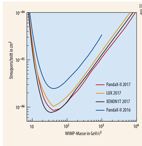
Abb. 1 XENONIT und PandaX-II liefern derzeit die größte Sensitivität bei der Suche nach WIMPs, wie sich an dem immer niedrigeren Streuquerschnitt zwischen WIMP und Atomkernen zeigt.
