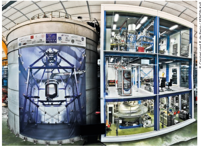
In einer der unterirdischen Hallen des Gran-Sasso-Labors steht der über zehn Meter hohe Tank mit dem XENONIT-Experiment.
