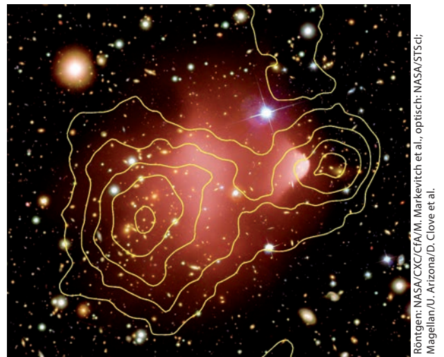
Abb. 2 Die Galaxien der Bullet-Haufen sind in dieser Hubble-Aufnahme in gelb/weiß gezeigt. Die meisten Baryonen befinden sich im Intracluster-Medium und leuchten im Röntgenlicht (Chandra-Aufnahme in rot). Dieses Gas wurde durch die Kollision komprimiert und abgebremst. Das zeigt sich an der namensgebenden „Bugwelle“ des rechten Haufens. Das Gravitationspotential der beiden Haufen wird von der Dunklen Materie dominiert (als Konturlinien gezeigt). Sie wechselwirkt nicht und hat sich daher (wie die Galaxien) von dem Röntgengas entfernt.
