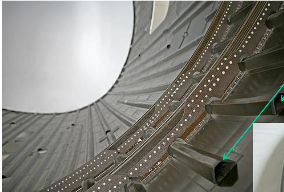
Geklebte CFK-Omega-Stringer (Boeing 787)
