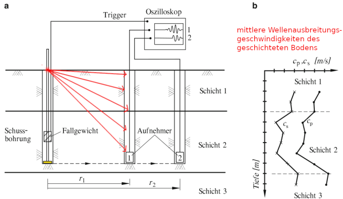
Abb. 23.19 Cross-Hole-Versuch, nach Empfehlungen „Baugrunddynamik“ (2002). a Prinzipielle Anordnung; b Wellen-Geschwindigkeitsprofil
