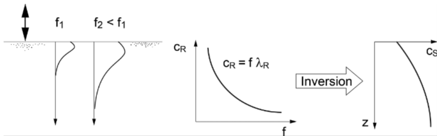
Bild 25 Ermittlung der Scherwellengeschwindigkeit aus Oberflächenwellenmessungen
