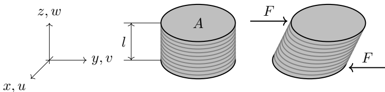
Abb. 2: Geometrie des Scherversuchs
