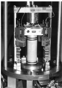
Bild 28 Resonant-Column-Versuch
