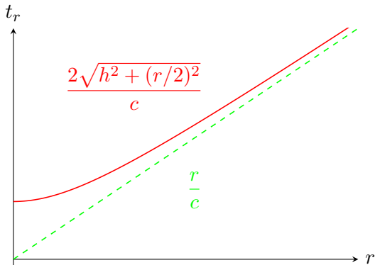
Wellenfade und Laufzeitdiagramm
