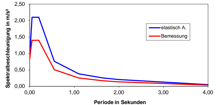
Antwortspektren für horizontale Anregung
