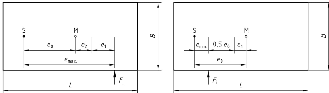
Bild 5 — Bestimmung der Exzentrizitäten der Horizontalkraft F_i
