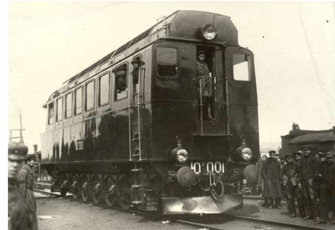
1923/24: Ee12 (Maschinenfabrik Esslingen) Gleichstrom-Gleichstrom – Übertragung, P_{DM} = 883 \text{ kW} , P_T = 800 \text{ kW}
