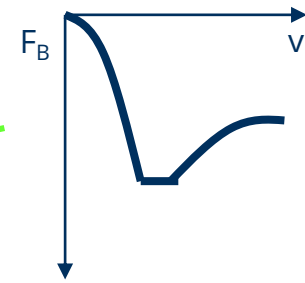
Retarder (Strömungsbremse)
