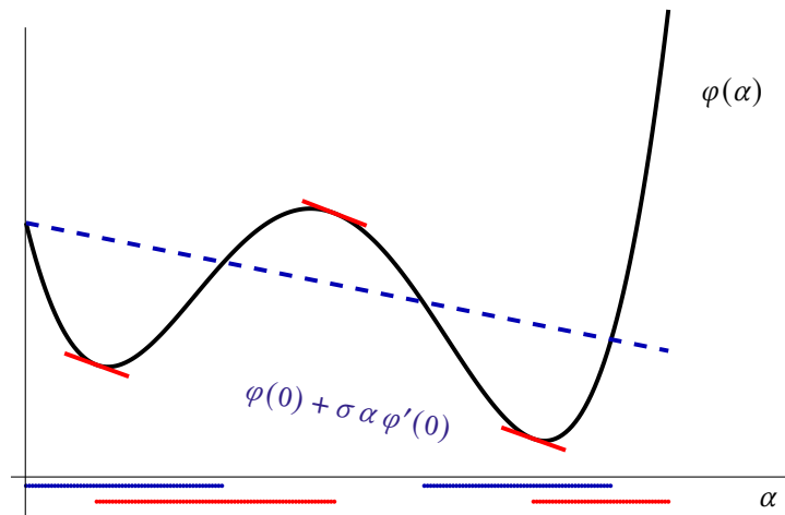
Abbildung 5.3: Illustration derjenigen Schrittweiten \alpha \geq 0 , die die Armijo-Bedingung (5.12) (blau) und die Krümmungsbedingung (5.16) erfüllen (rot). Als Parameter sind hier \sigma = 0.05 und \tau = 0.1 gewählt.
