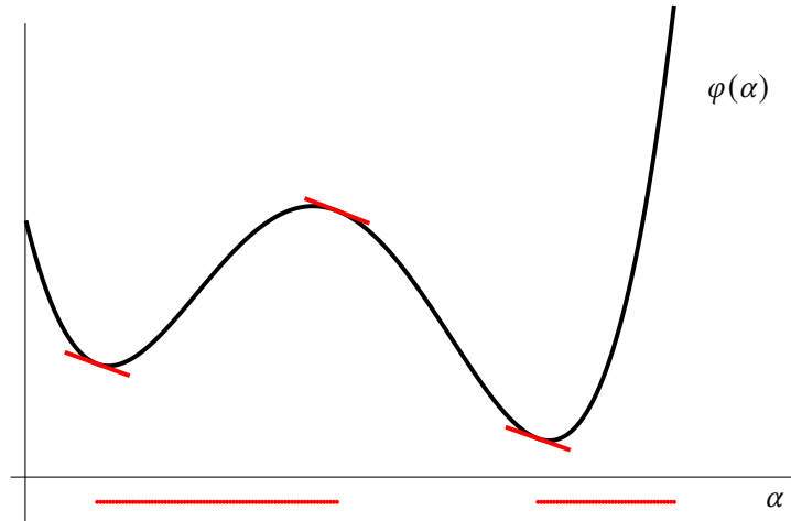
Abbildung 5.2: Illustration derjenigen Schrittweiten \alpha \geq 0 , die die Krümmungsbedingung (5.16) erfüllen (rot). Als Parameter ist hier \tau = 0.1 gewählt.
