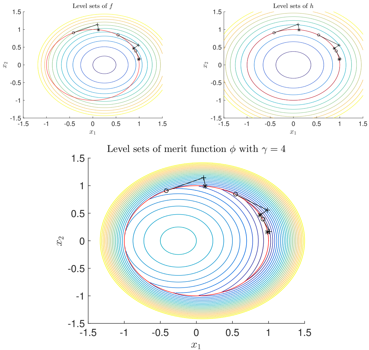
Abbildung 11.1: Contour-Plots der Zielfunktion (oben links), der Gleichungsnebenbedingung (oben rechts) und der Merit-Funktion (unten) für das Beispiel zum Maratos-Effekt. Der rote Kreis markiert die zulässige Menge. Weiterhin sind drei Iterierte ( \circ ), der volle SQP-Schritt (+) und der second-order-correction-Schritt (*) dargestellt.
