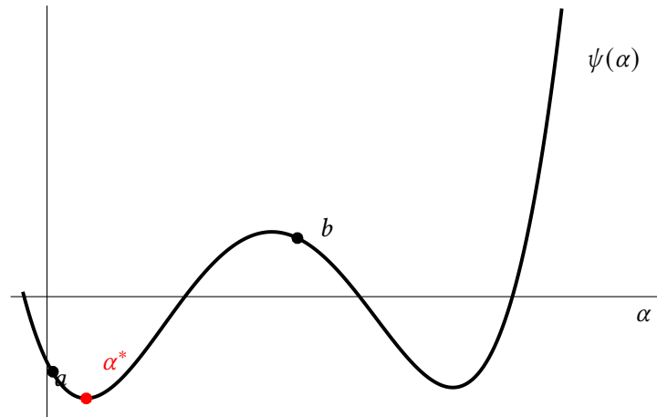
Abbildung 5.4: Illustration der Bedingung (5.18) und der Aussage von Lemma 5.15.
