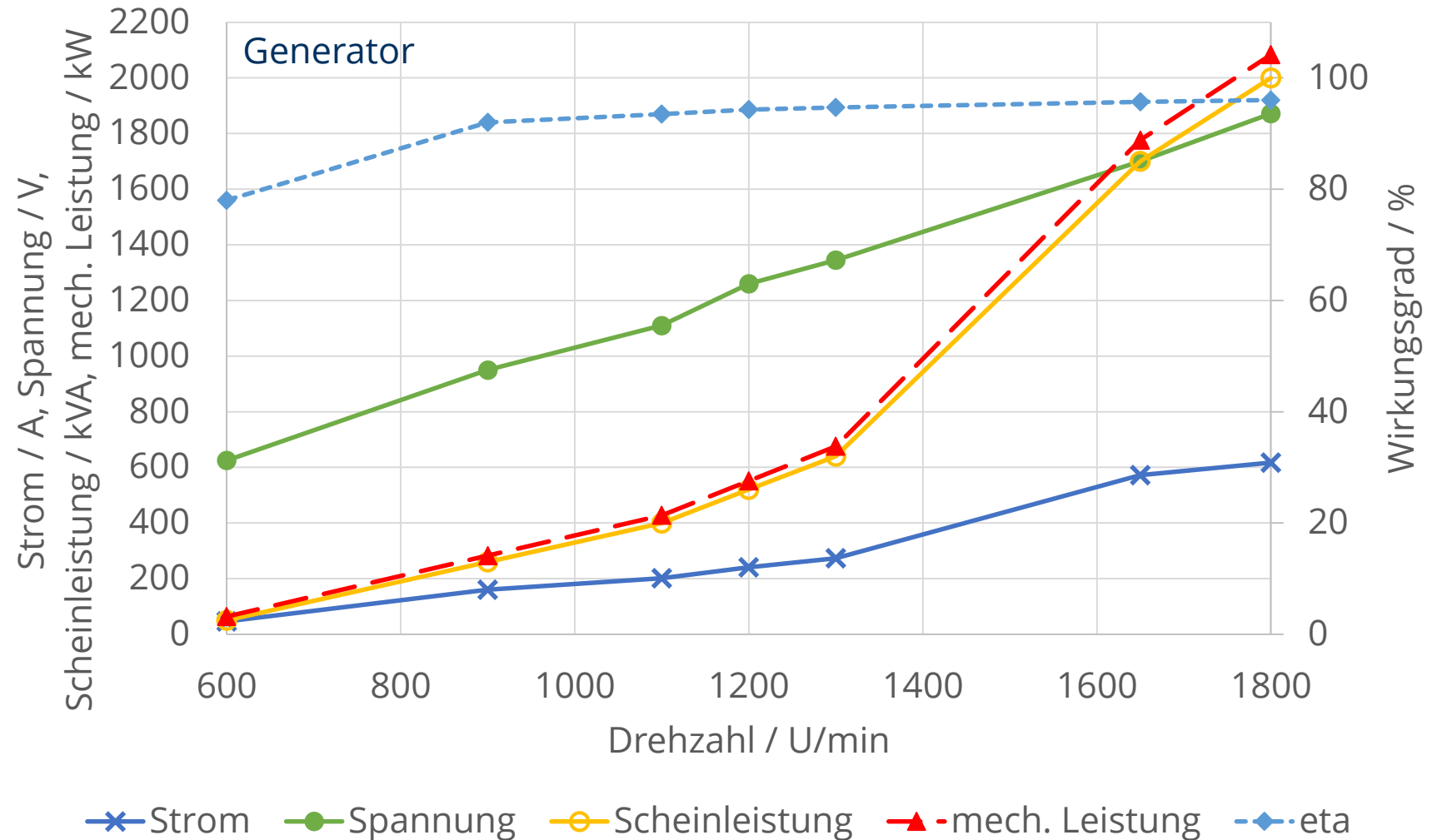
Siemens ER 20 / ÖBB Rh 1616
