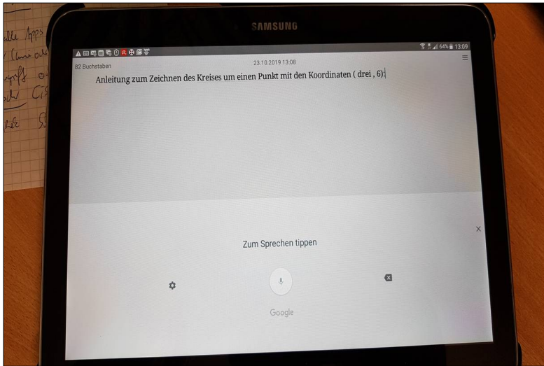
„WriterP“ (Android)
