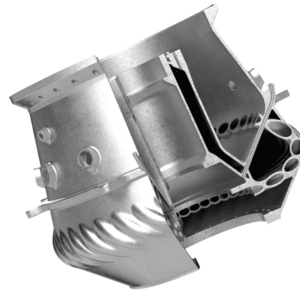
Turbinenbauteil (Ø560x427mm, 120kg, In718, 69h)
