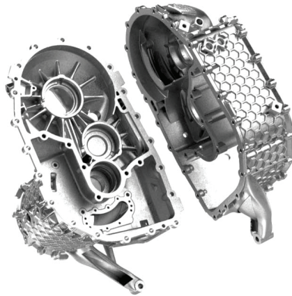
Motorgehäuse (590x560x367mm, 15,5kg, AlSi10Mg, 21h)
