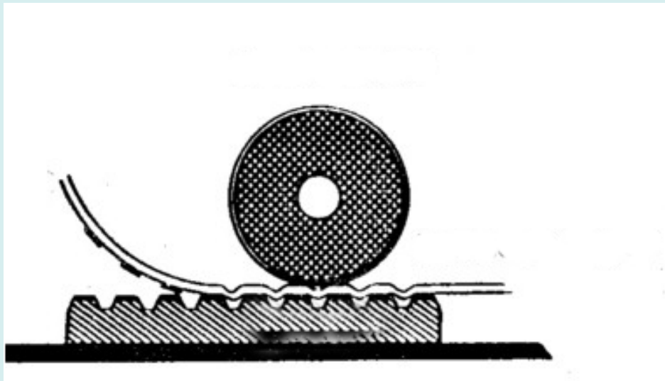
Zylinder gegen Fläche (Schnellpresse)
