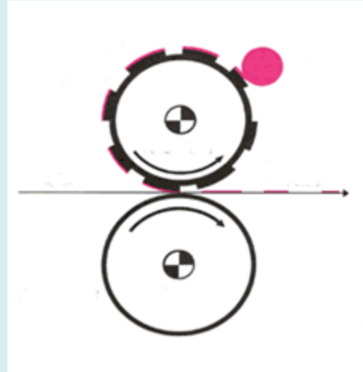
Zylinder gegen Zylinder (Rotationsmaschine)
