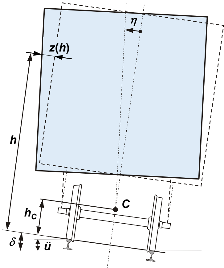
Fahrt auf überhöhtem Gleis mit Überhöhungsfehlbetrag
